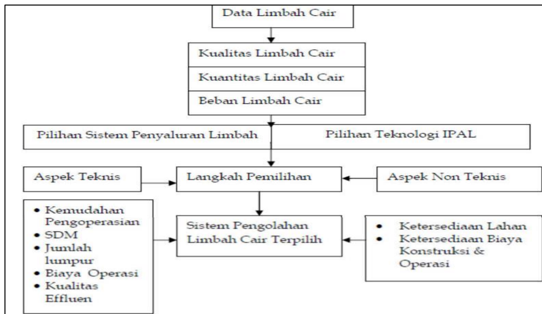
Gambar 4.24 Bagan Alir Pemilihan Unit Pengolahan pada IPAL
