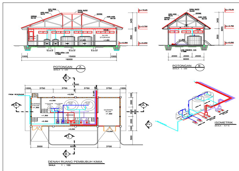
Gambar 3.7 Gambar Tipikal Bangunan Kimia IPA
