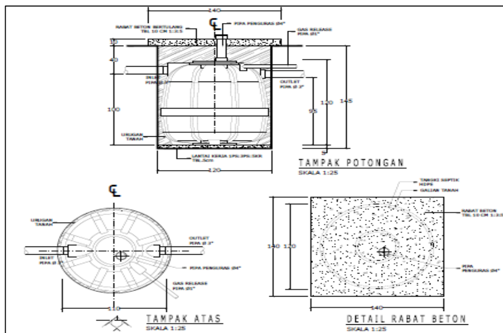
Gambar 4.19 Tangki Pabrikan
